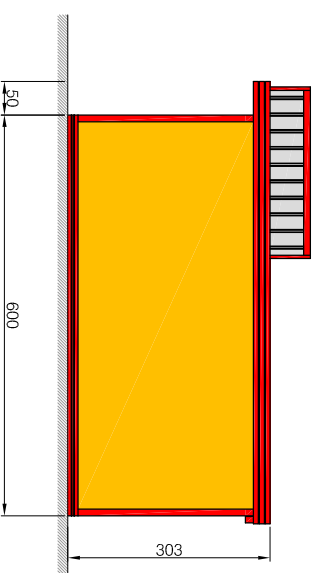
PROSPETTO LATERALE
