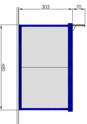
PROSPETTO LATERALE
