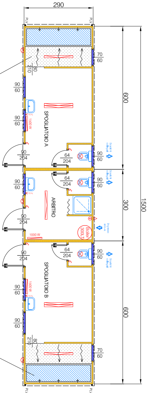
PIANTA
