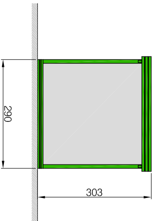
PROSPETTO LATERALE
