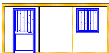
PROSPETTO PRINCIPALE SPECIAL 500 X 240 X H 240
