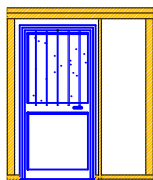
PROSPETTO PRINCIPALE SPECIAL 200 X 200 (240) X H 240
