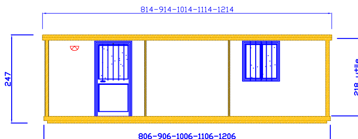
PROSPETTO PRINCIPALE CANTIERE 806-906-1006-1106-1206 X 240 X H 240
