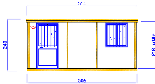
PROSPETTO PRINCIPALE CANTIERE 506 X 240 X H 240
