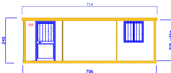
PROSPETTO PRINCIPALE CANTIERE 706 X 240 X H 240
