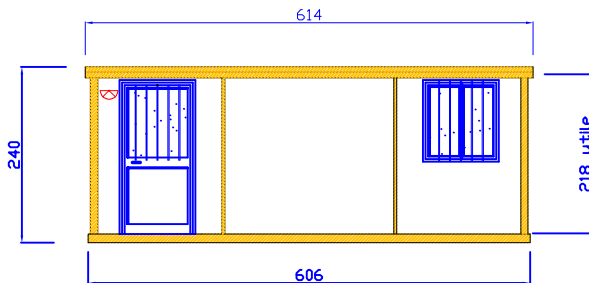
PROSPETTO PRINCIPALE CANTIERE 606 X 240 X H 240
