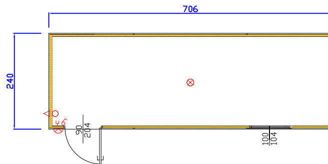
CANTIERE 706 X 240 X H 240
