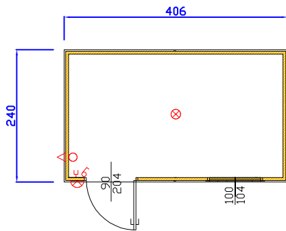
CANTIERE 406 X 240 X H 240
