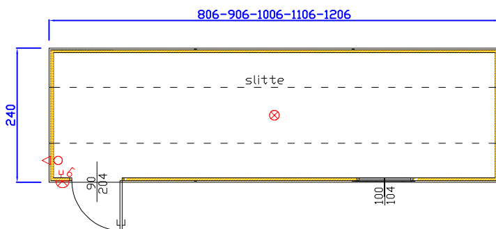
CANTIERE 806-906-1006-1106-1206 X 240 X H 240
