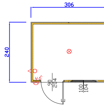
CANTIERE 306 X 240 X H 240
