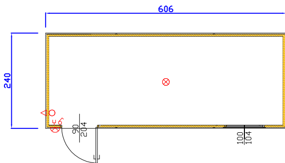
CANTIERE 606 X 240 X H 240
