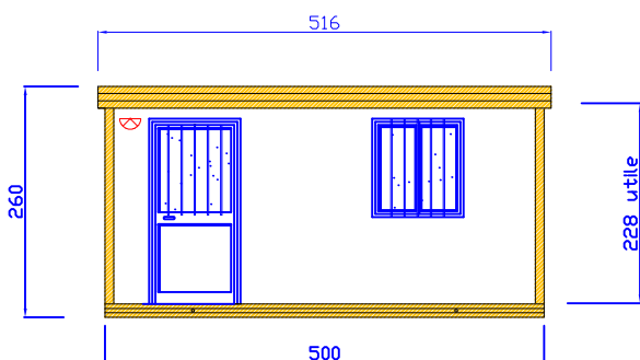
PROSPETTO PRINCIPALE STANDARD 500 X 240 X H 260
