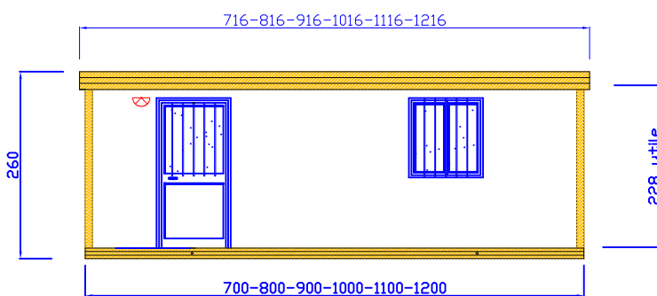
PROSPETTO PRINCIPALE STANDARD 700-800-900-1000-1100-1200 X 240 X H 260
