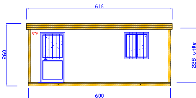
PROSPETTO PRINCIPALE STANDARD 600 X 240 X H 260
