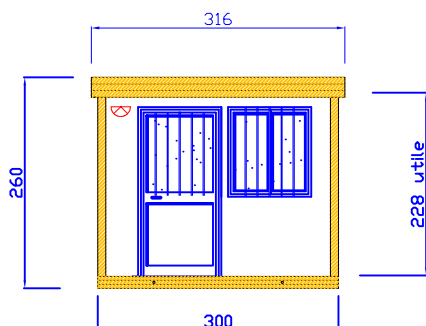
PROSPETTO PRINCIPALE STANDARD 300 X 240 X H 260
