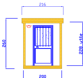
PROSPETTO PRINCIPALE STANDARD 200 X 240 X H 260
