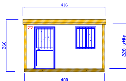
PROSPETTO PRINCIPALE STANDARD 400 X 240 X H 260
